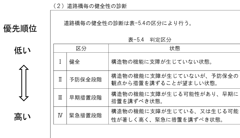
図-3 健全性による優先順位
