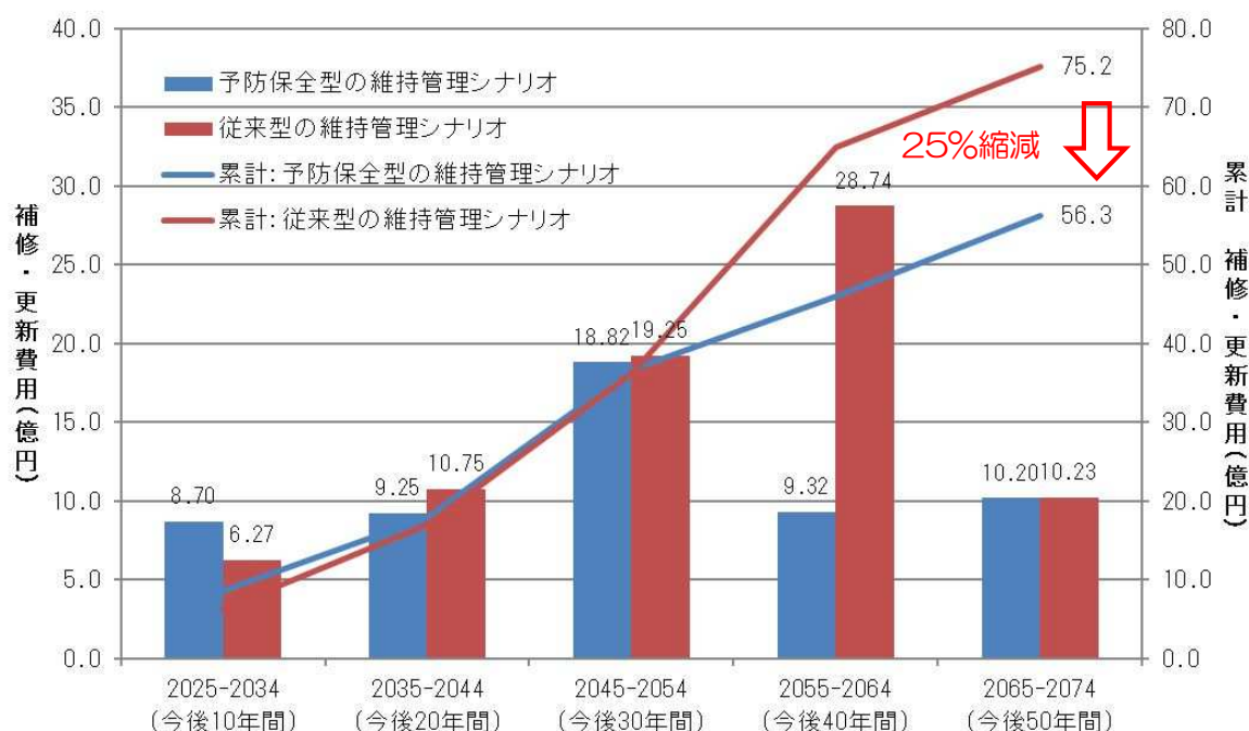
図-4 今後50年の維持管理コストの比較
